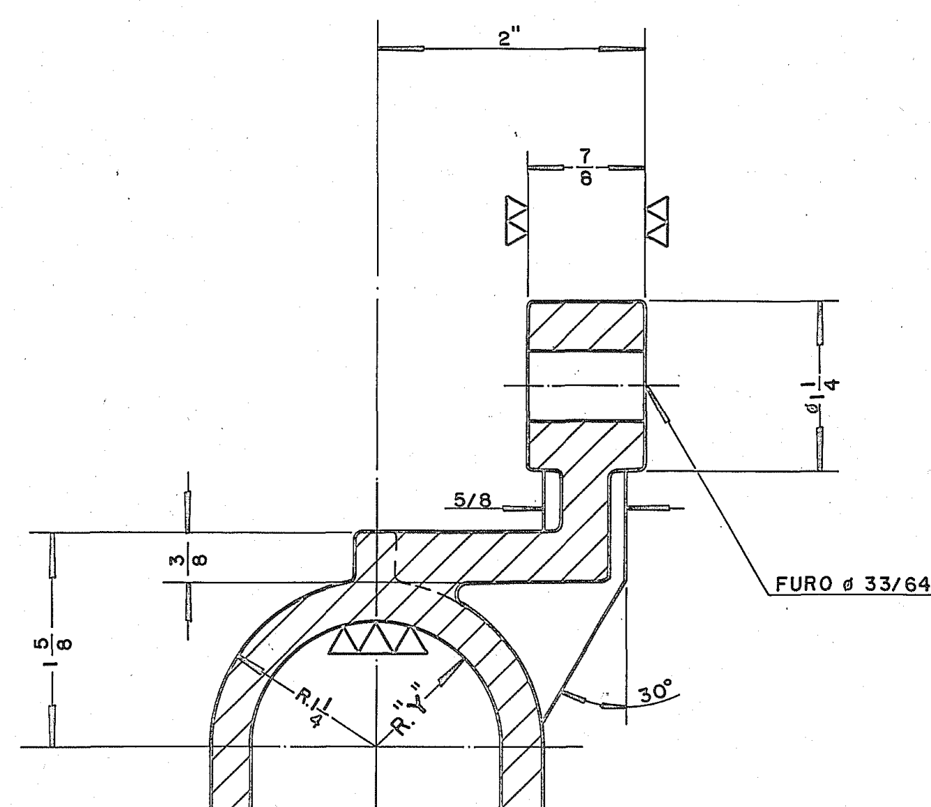
CORTE CC
