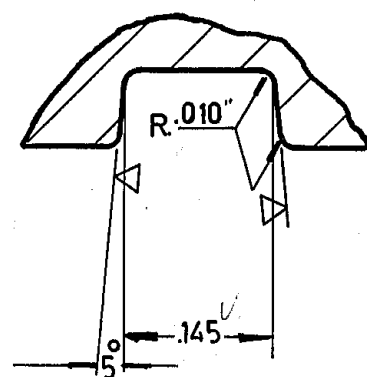
DETALHE "A" ESC. 5:1
