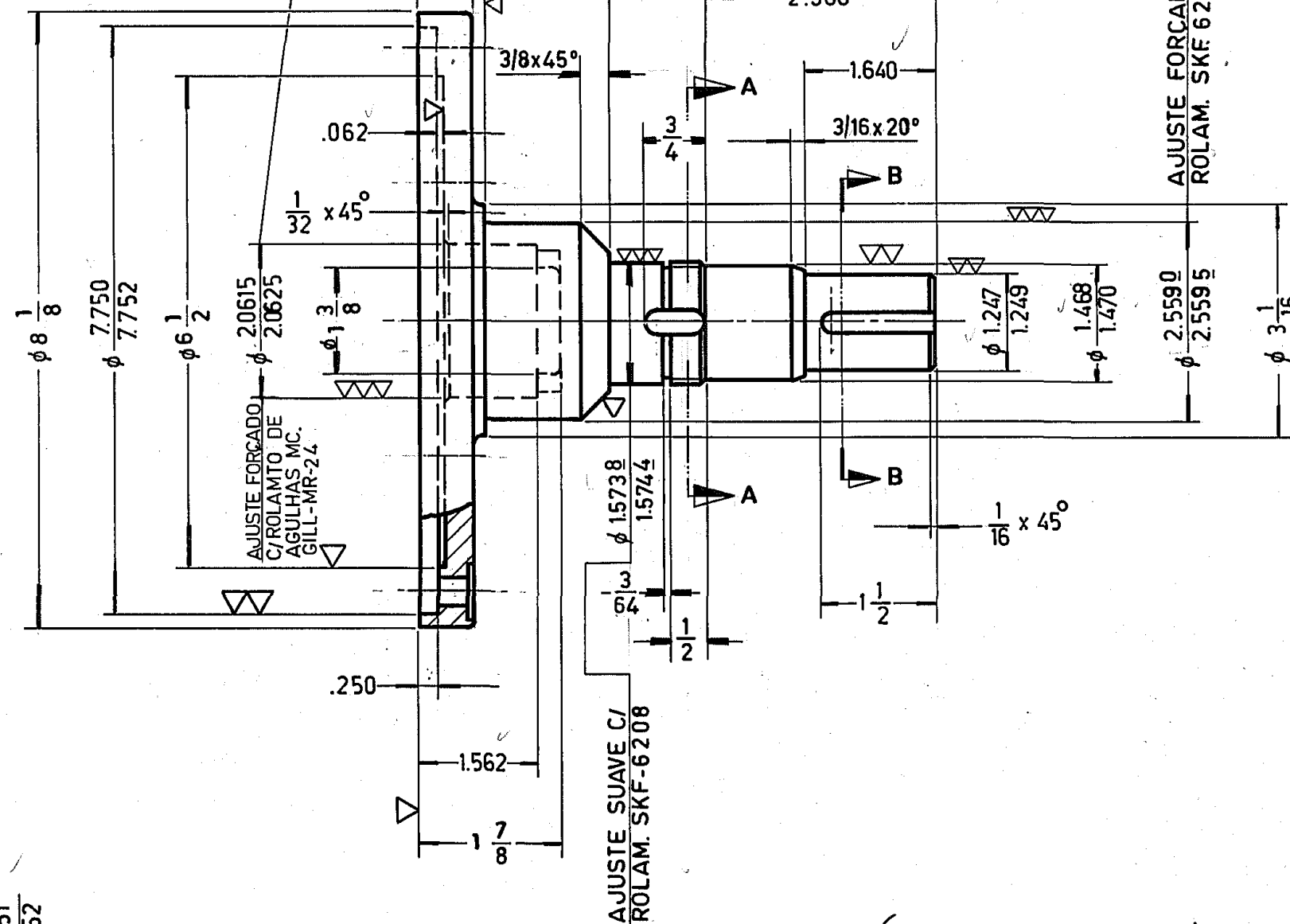
DETALHE DO FUNDO NO FURO DO ROLAMENTO
