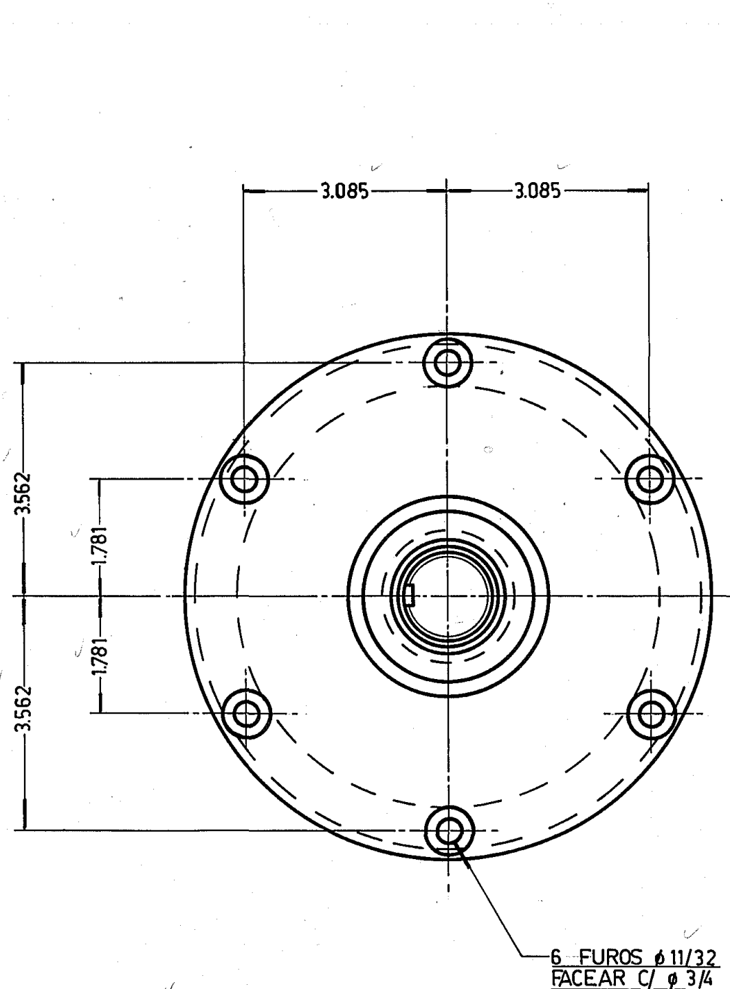
DETALHE DO FUNDO NO FURO DO ROLAMENTO
