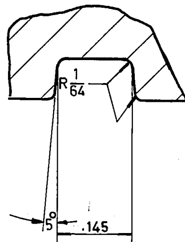
DETALHE "A" ESC. 5:1
