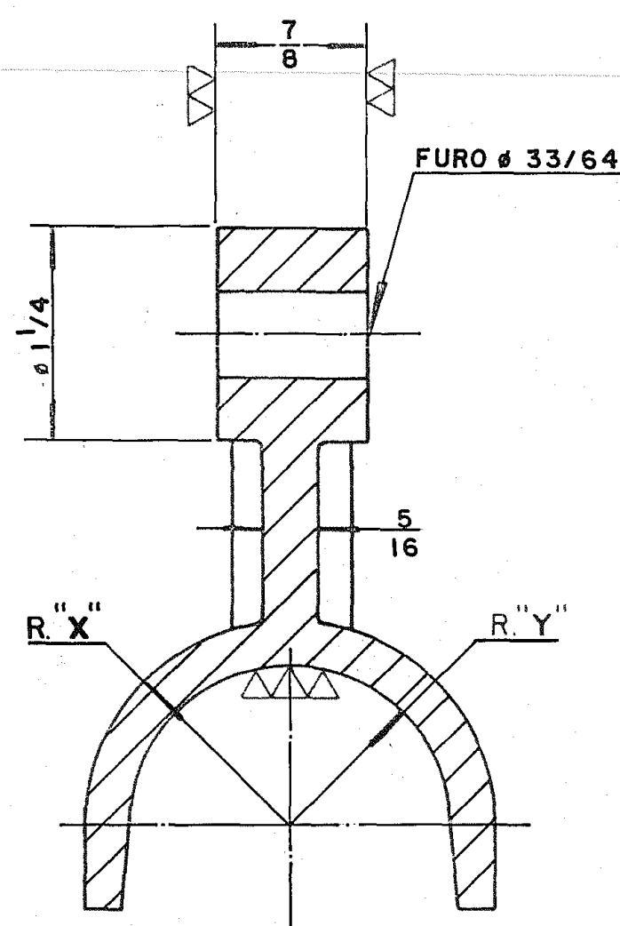
CORTE AA
