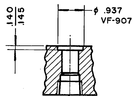
SEÇÃO B-B
