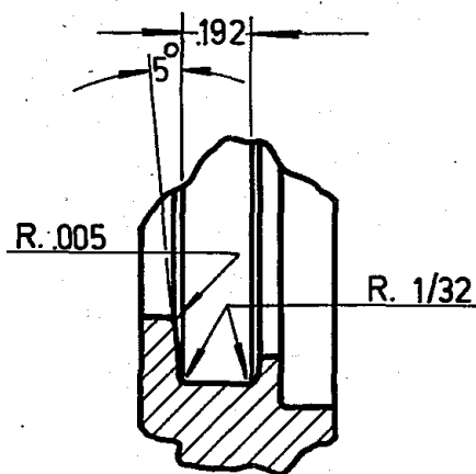
DETALHE "A" ESC. 2:1
