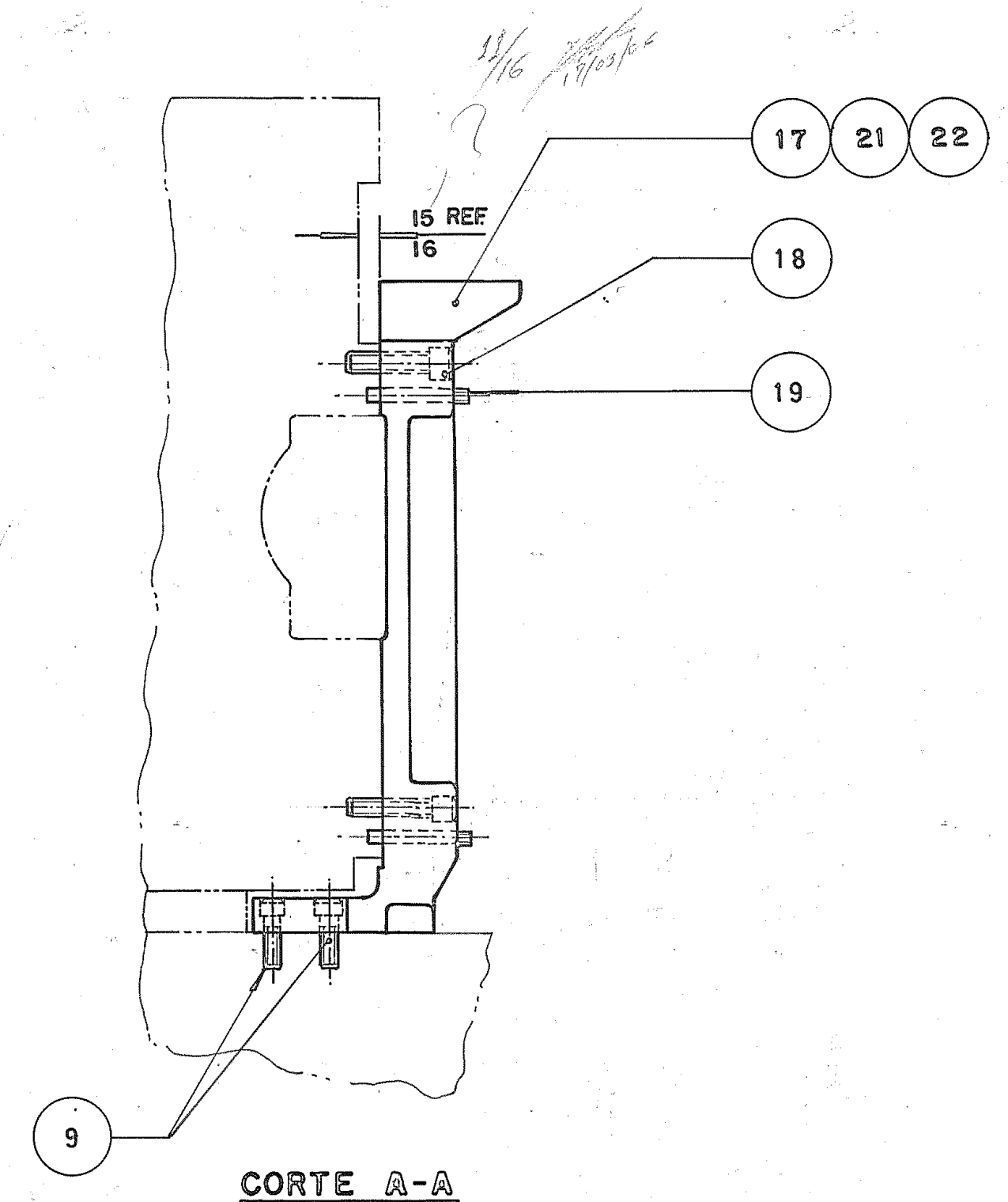
CORTE A-A DETALHE DO SUPORTE PARA CAIXA DE VÁLVULA ELETR. ESC. 1/4
