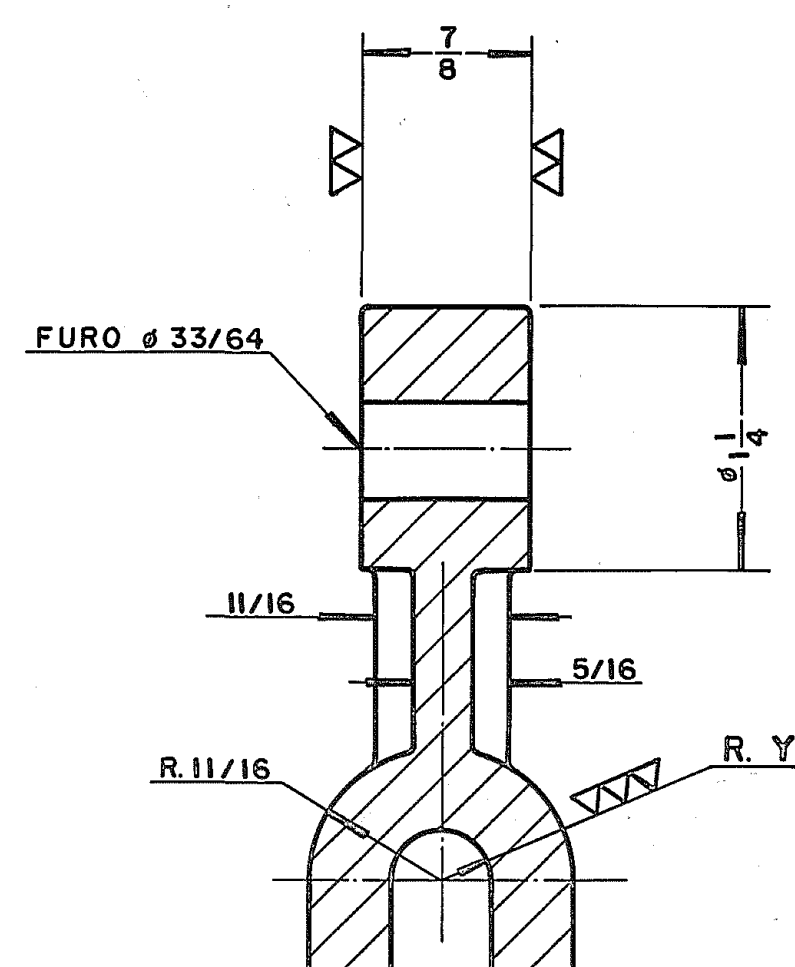
CORTE CC
