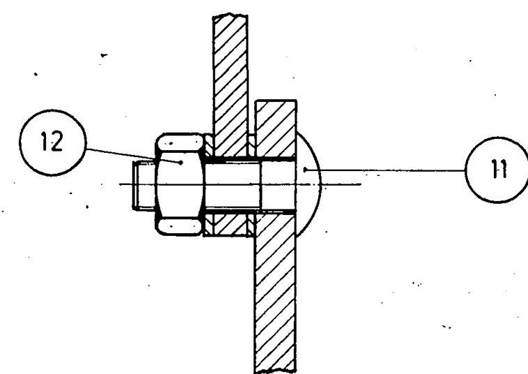
DETALHE A ESCALA 1:1
