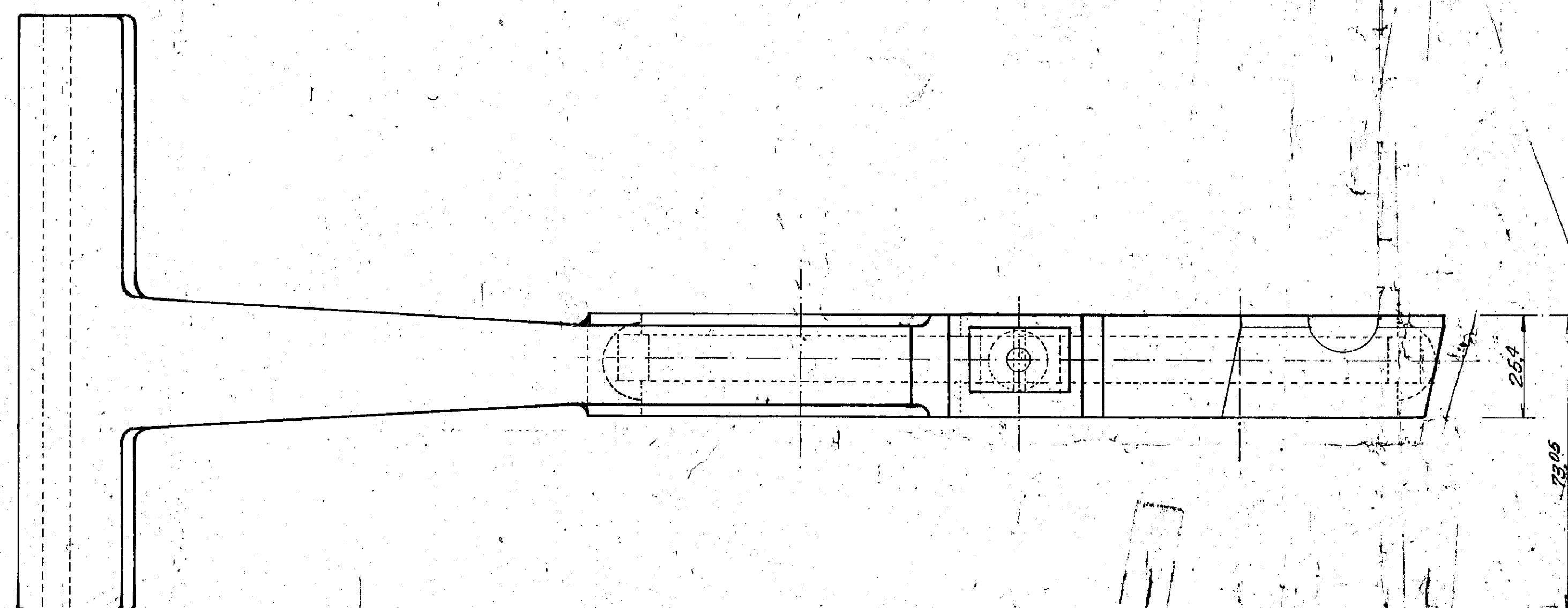
PLANTA E CORTE-BB
