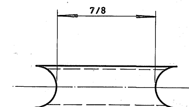
DETALHE DA PEÇA POS. 5 ESC.: 2:1
