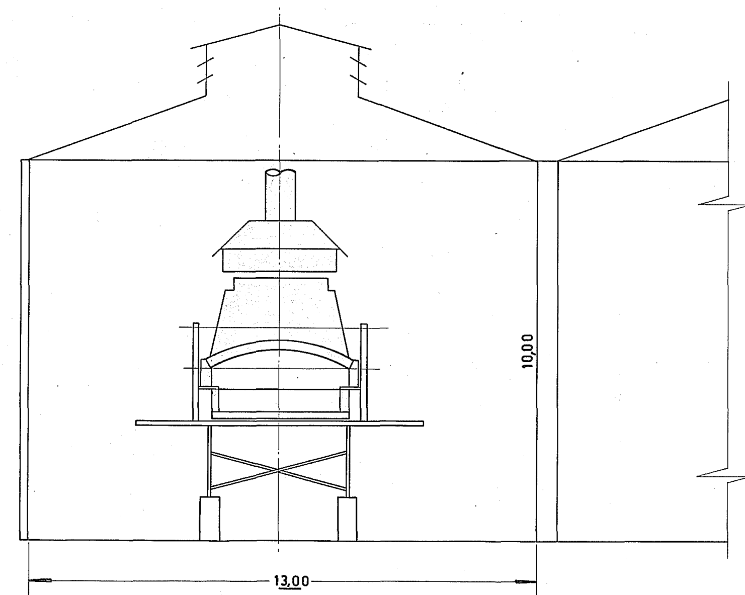
CORTE B-B
