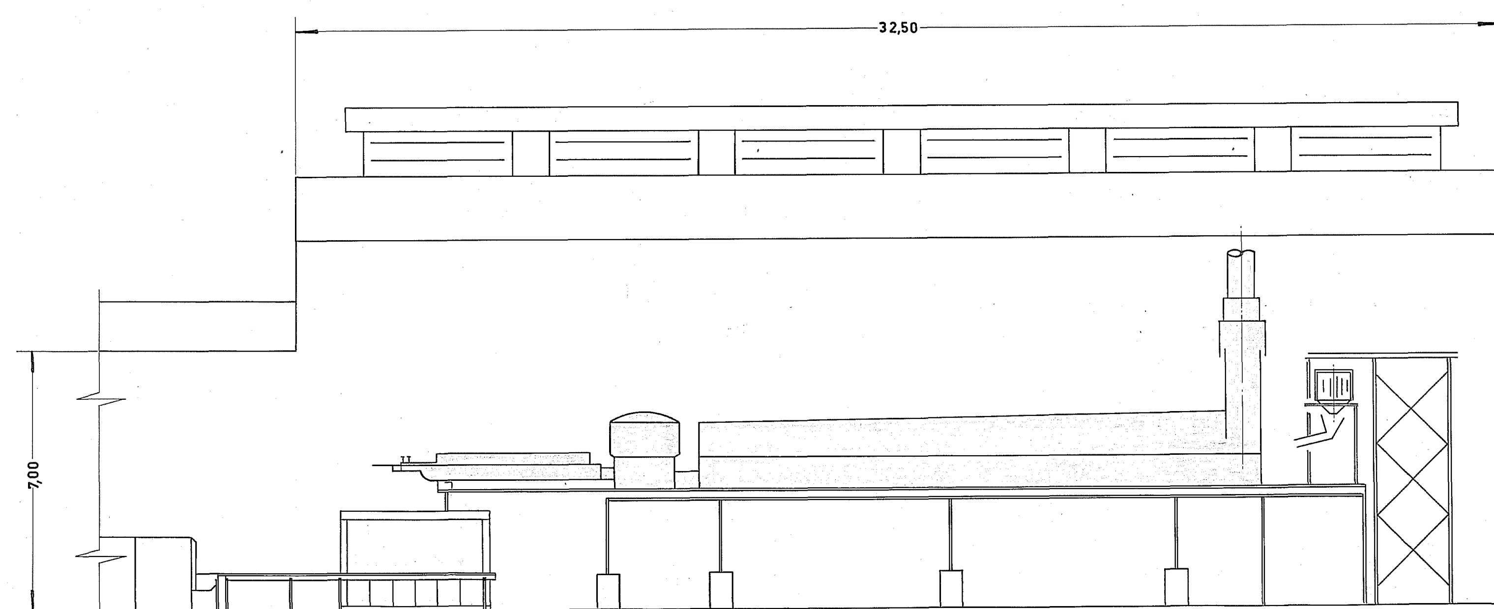
CORTE A-A
