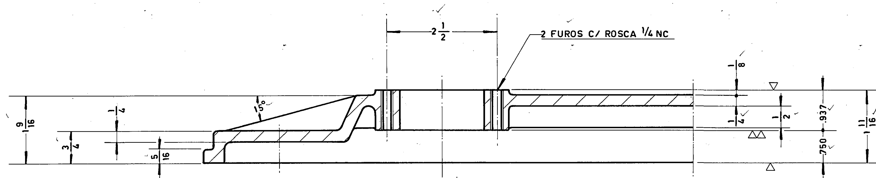
CORTE A-A
