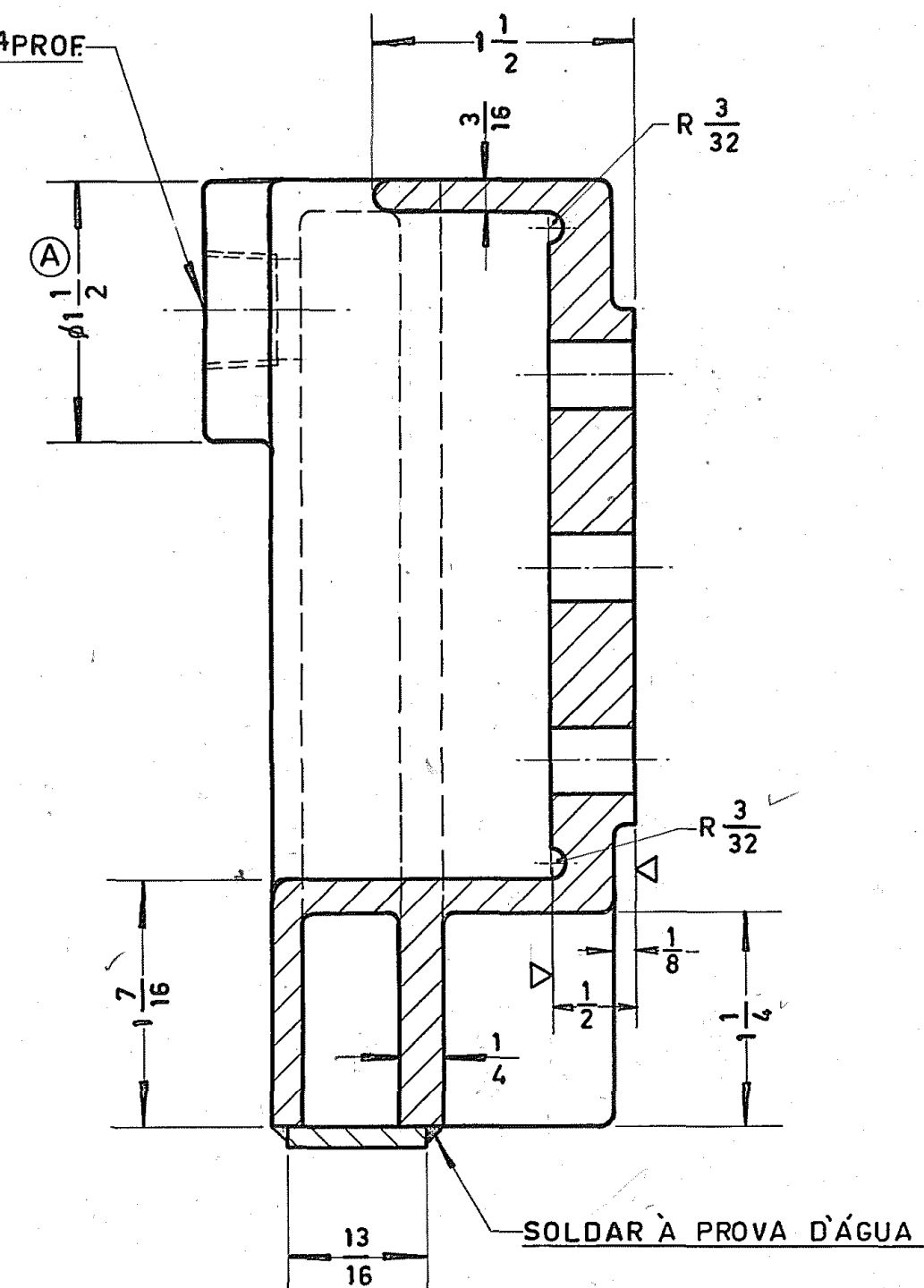
CORTE A-A
