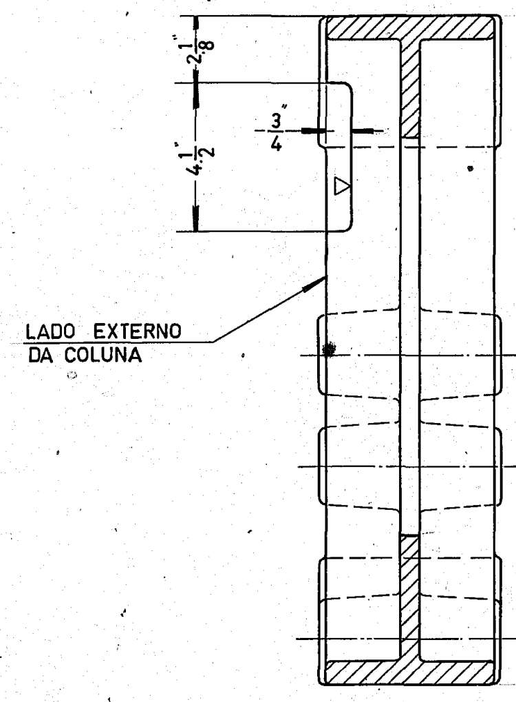
SEÇÃO-AA ESC. 1/4
