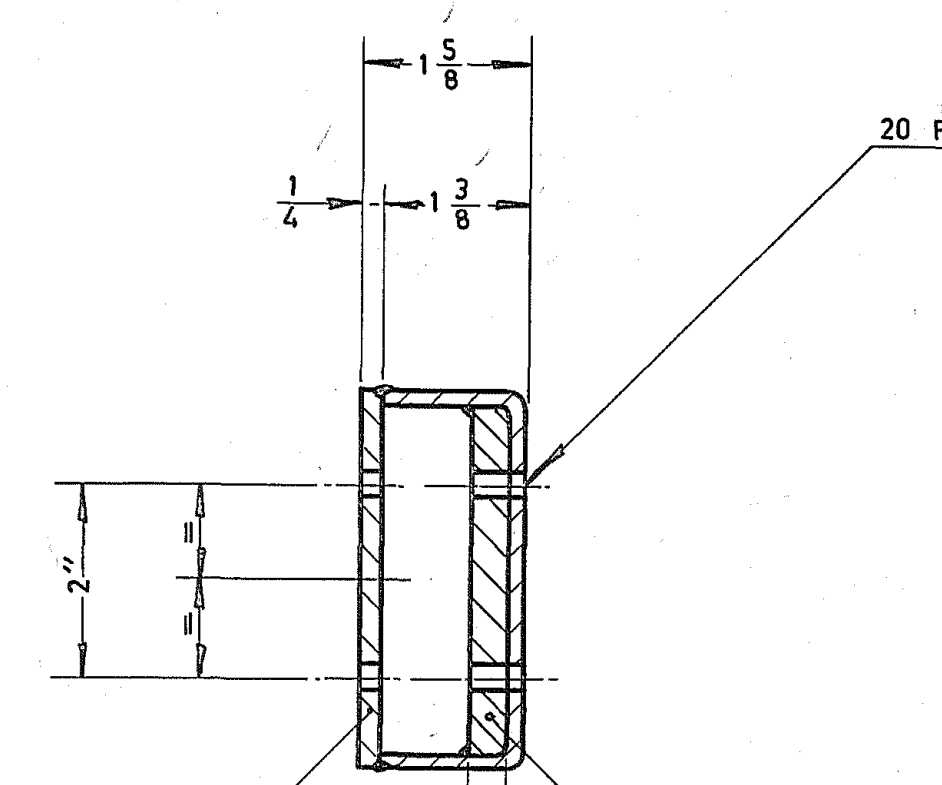
AÇO SAE 1020 (2 PEÇAS)
