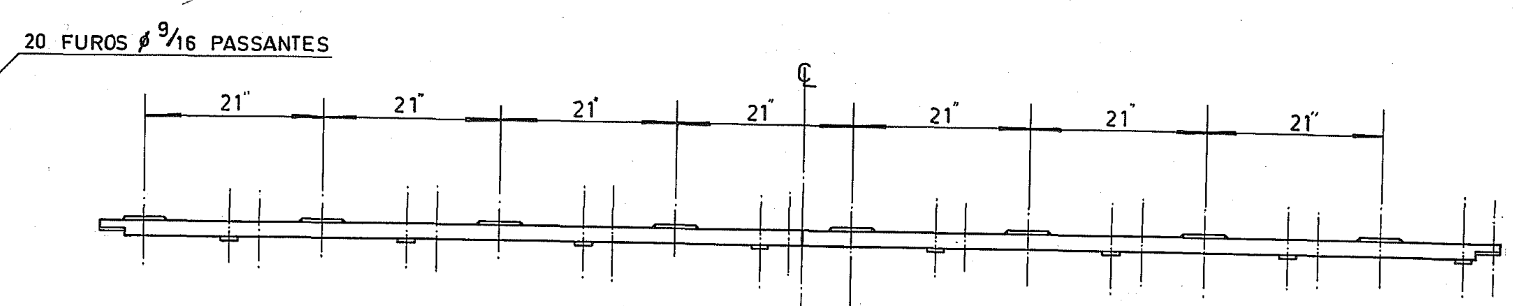
DETALHE Y ESC.: 1/16
