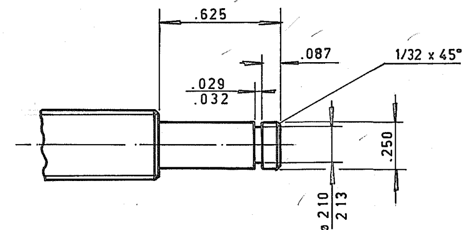
DETALHE W ESCALA: 2:1
