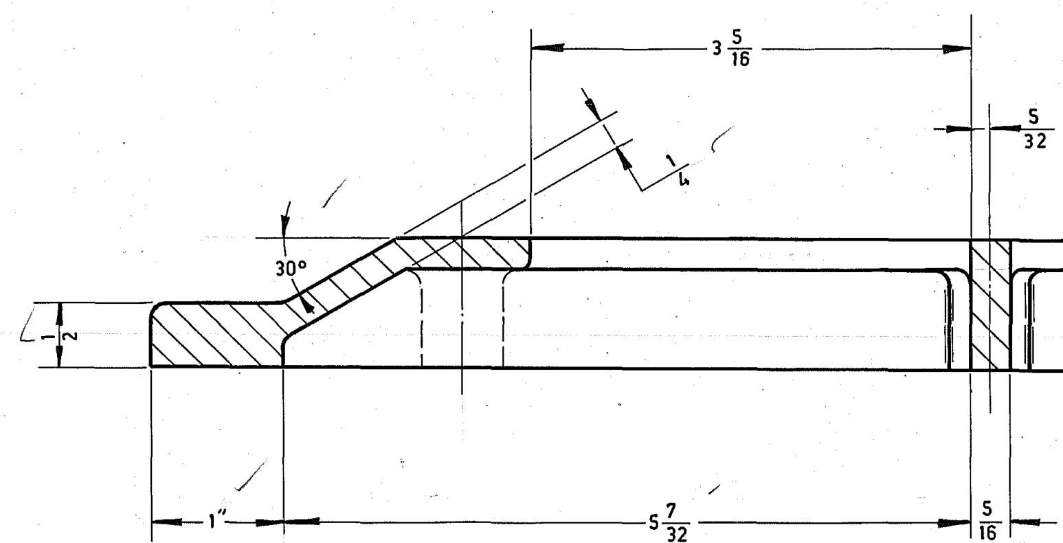
CORTE A-A
