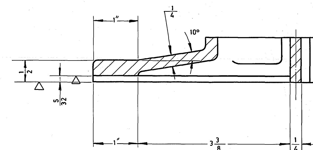
CORTE B-B
