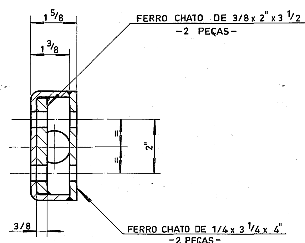
CORTE-CC ESC.: 1:2
