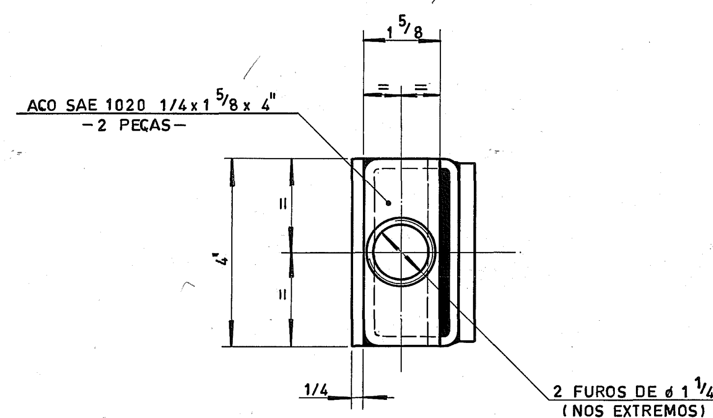
VISTA-A ESC.: 1:2
