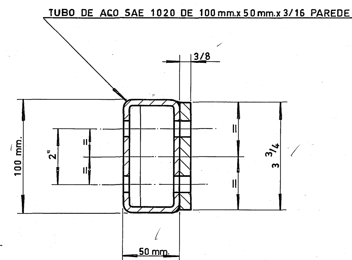
CORTE-BB ESC.: 1:2
