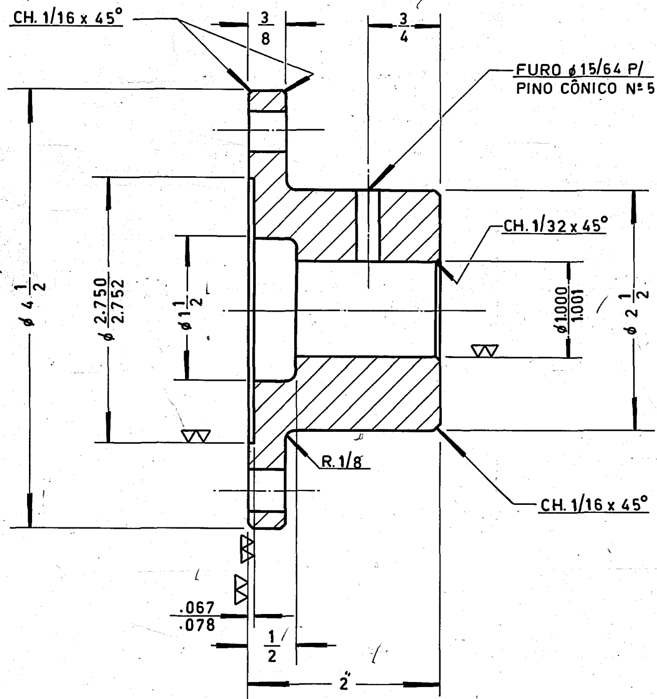
CORTE A-A
