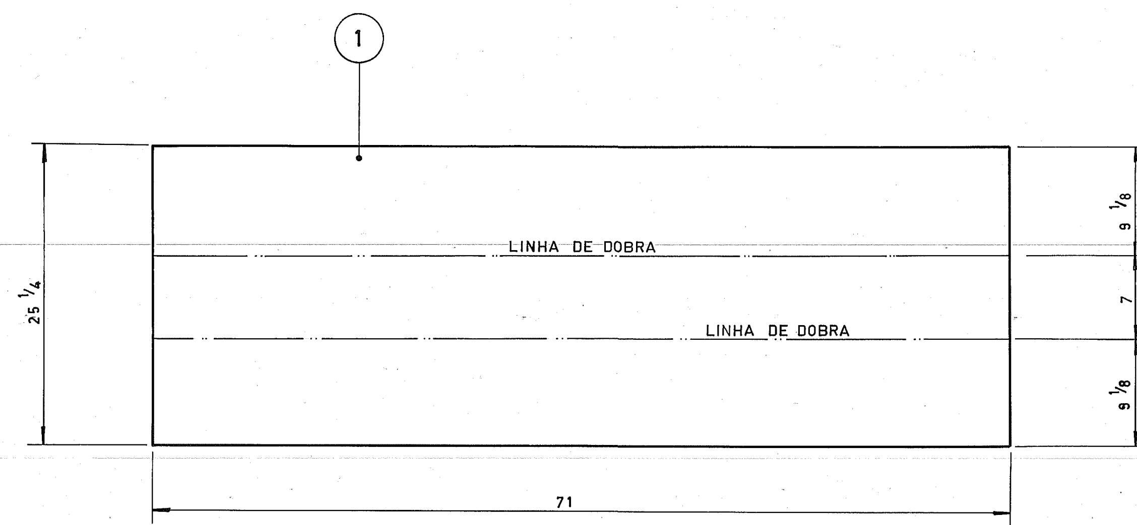
PEÇA DESENVOLVIDA ESCALA : 1/8
