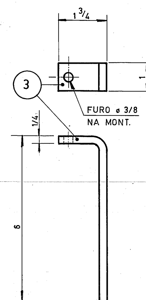
ESC. 1/2 DETALHE 3 QUANT. 2 pçs
