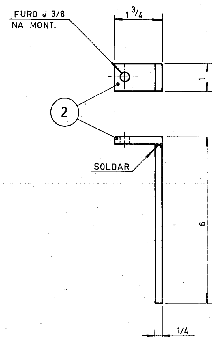
ESC. 1/2 DETALHE 2 QUANT. 2 pçs
