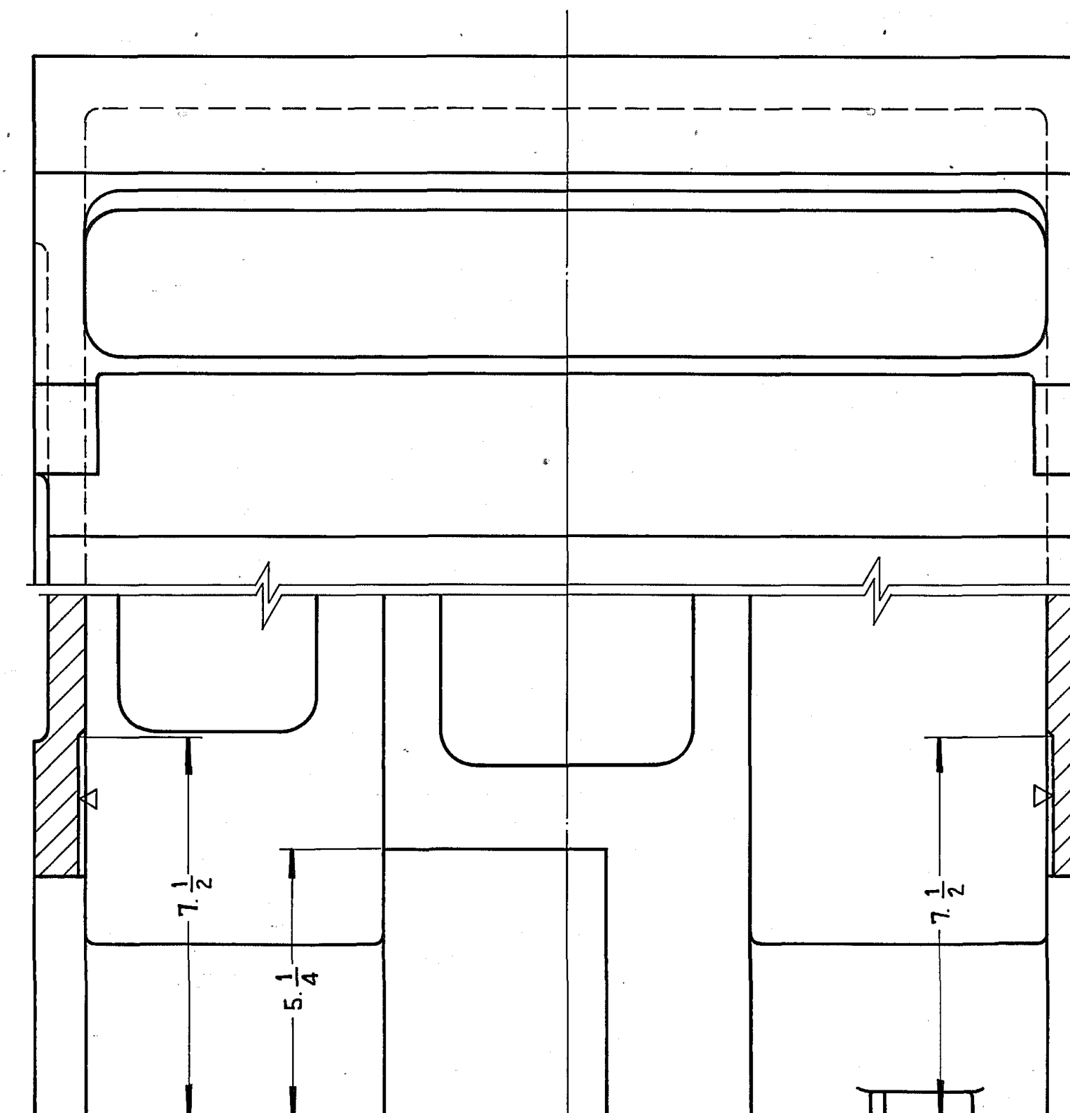
CORTE PARCIAL "AA"
