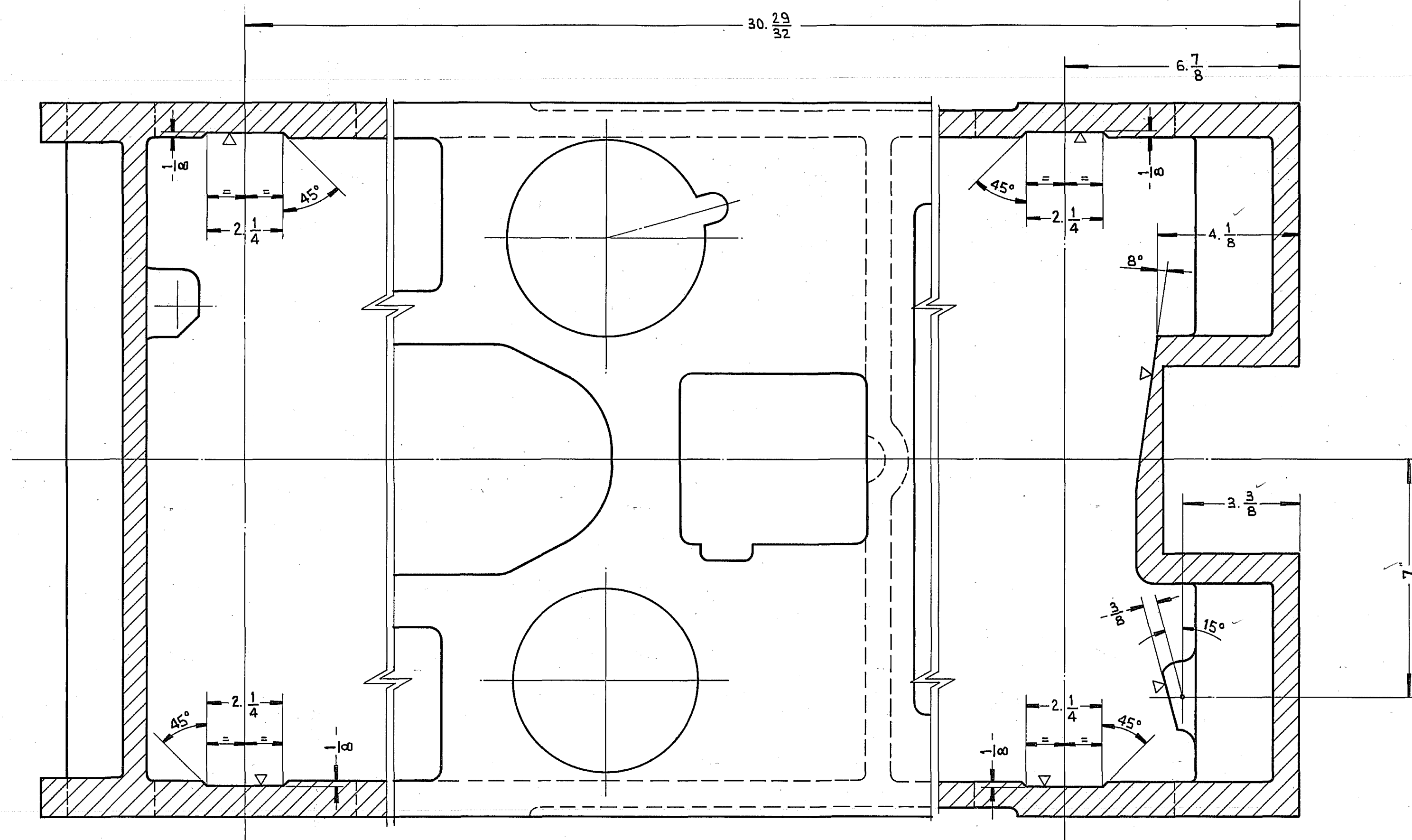
CORTE PARCIAL "BB"
