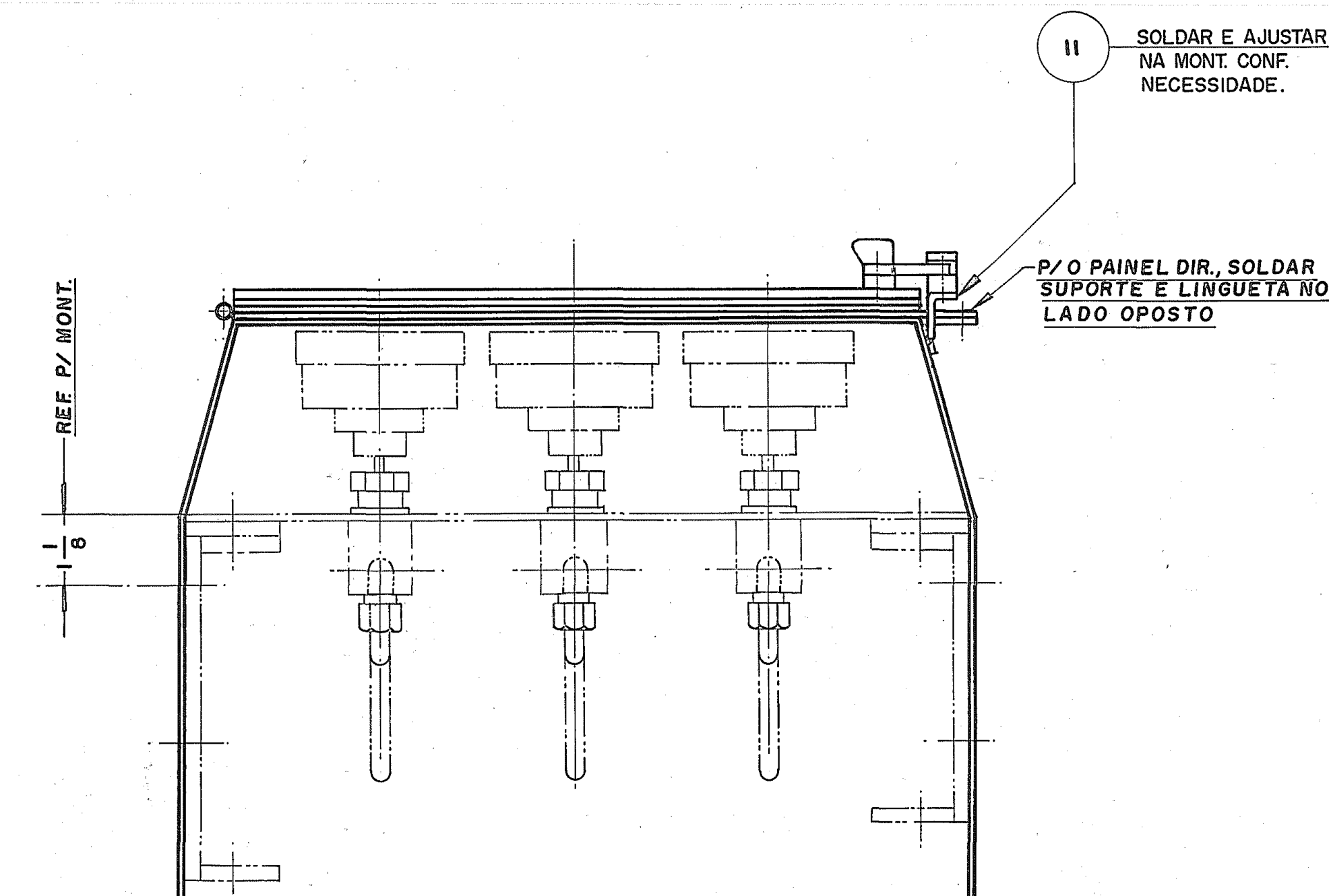
VISTA DE TÔPO (PAINEL ESQ.)
