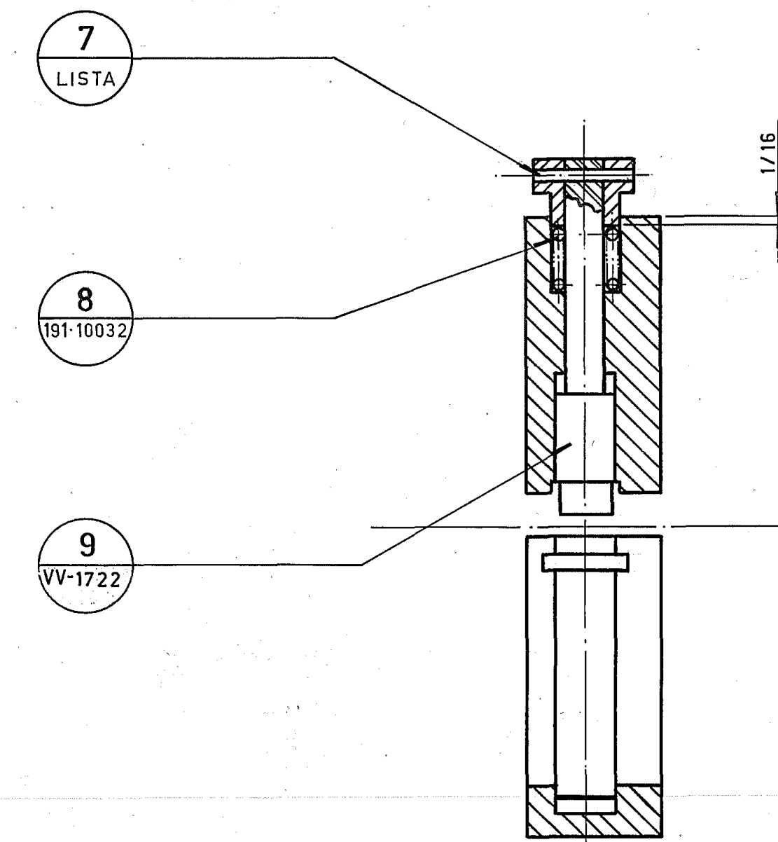
CORTE A-A
