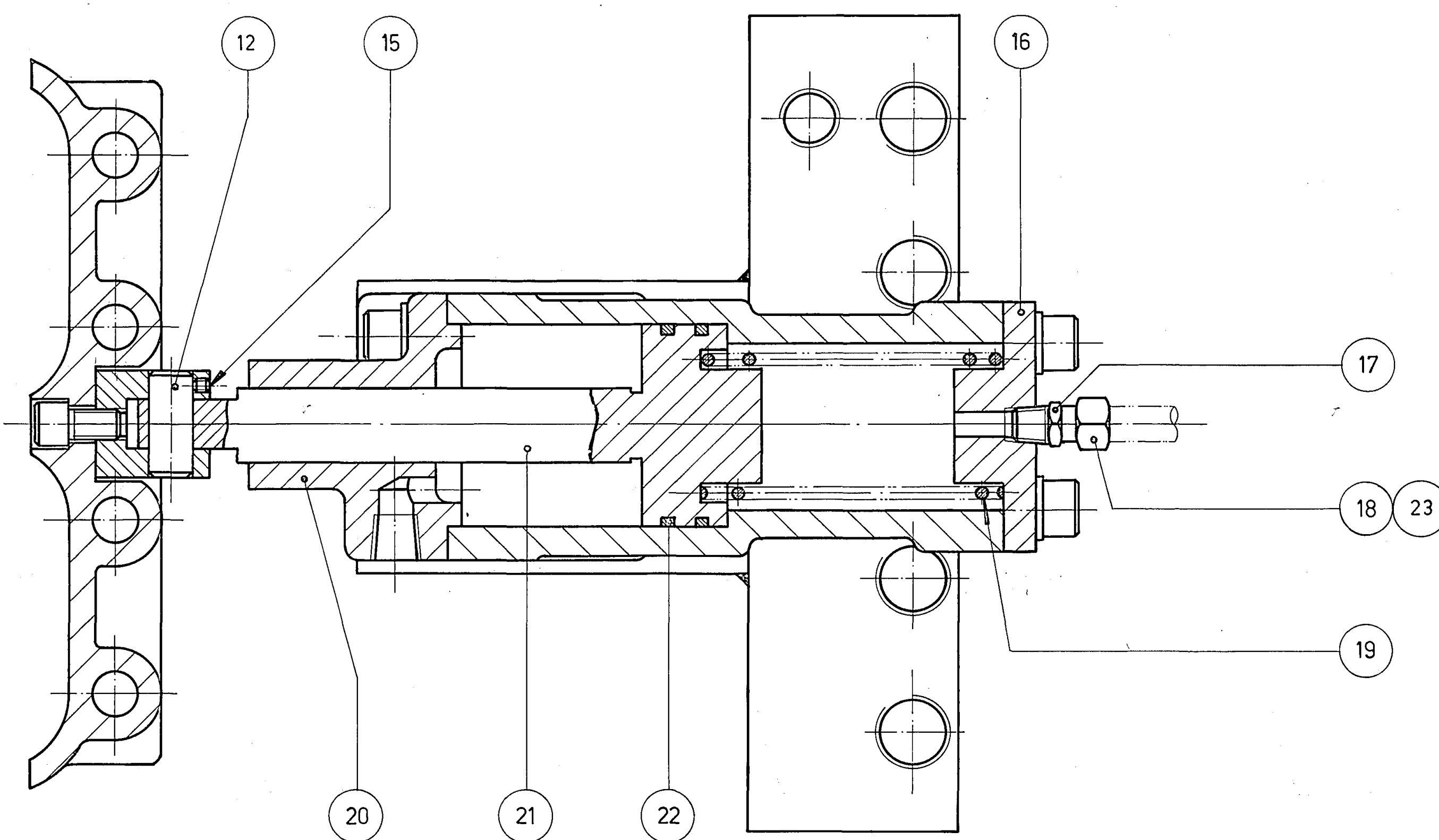
CORTE A-A
