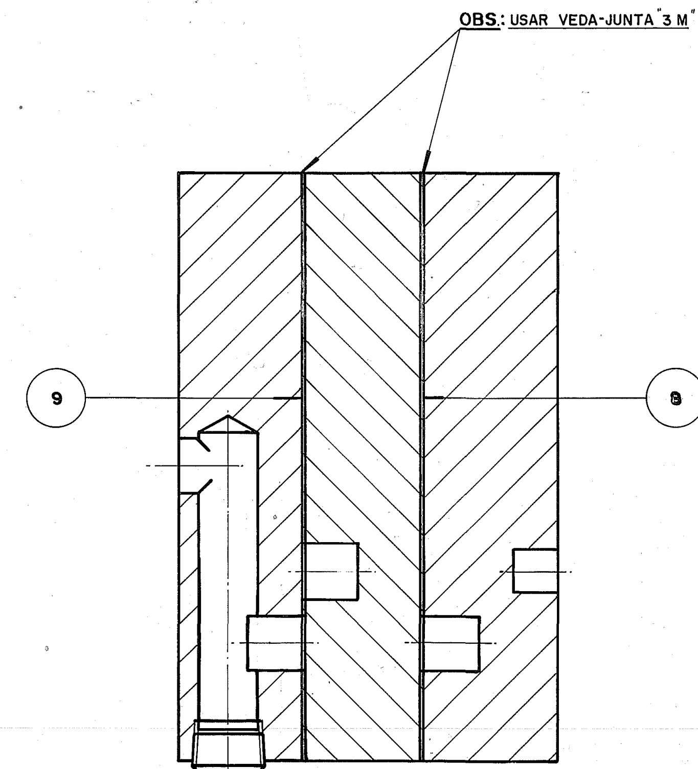
CORTE A - A POS. 16 (PLACA 19 POS.)
