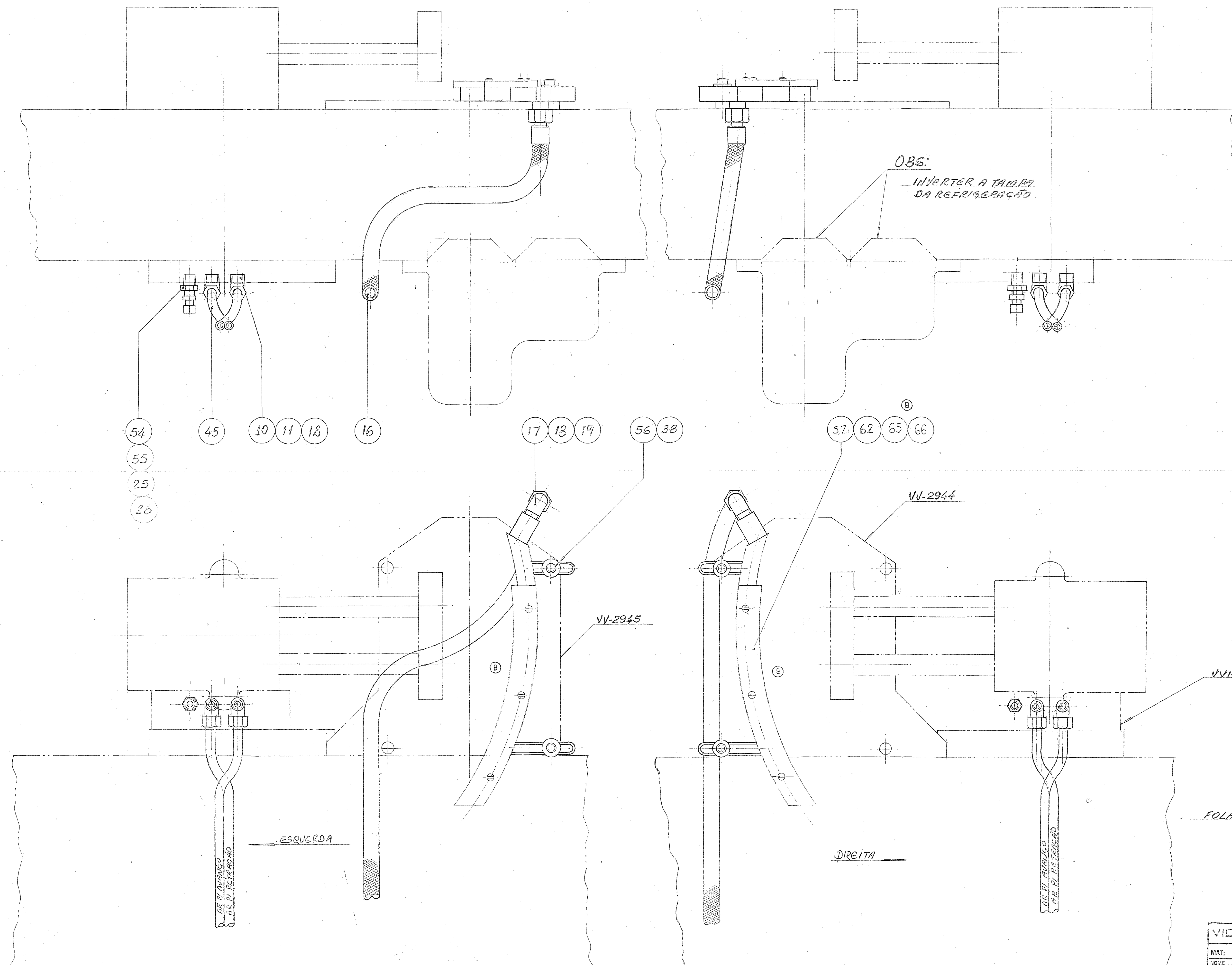
MONTAGEM DO PUXADOR PI ESTEIRA TRAB. A ESQUERDA
