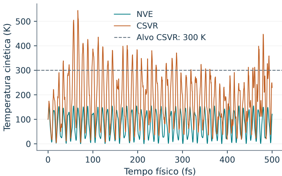
Figura 2.1: Par água XTB2, 0–500 fs: temperatura instantânea em NVE e com CSV. A referência de 300 K pertence somente ao caso termostatizado.
