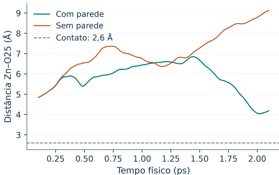
Figura 7.1: Zn–O25 nos dois controles XTB2/ALPB/CSV. O relógio da continuação vai até 2,1 ps; O25 já pertence à camada externa.
