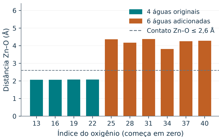
Figura 6.1: Geometria estática do solvato XTB2/ALPB: distâncias Zn-O das águas originais e acrescentadas. O corte de 2,6 Å identifica a primeira camada pelo critério do curso.
