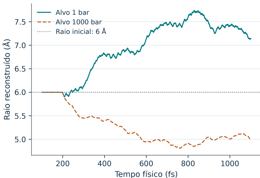
Figura 10.1: C2, XTB2/ALPB(water), CSVr a 300 K. Raio reconstruído da densidade registrada, com massa constante e raio inicial de 6 Å. A linha pontilhada marca o raio inicial; o eixo usa o relógio preservado pelo restart.
