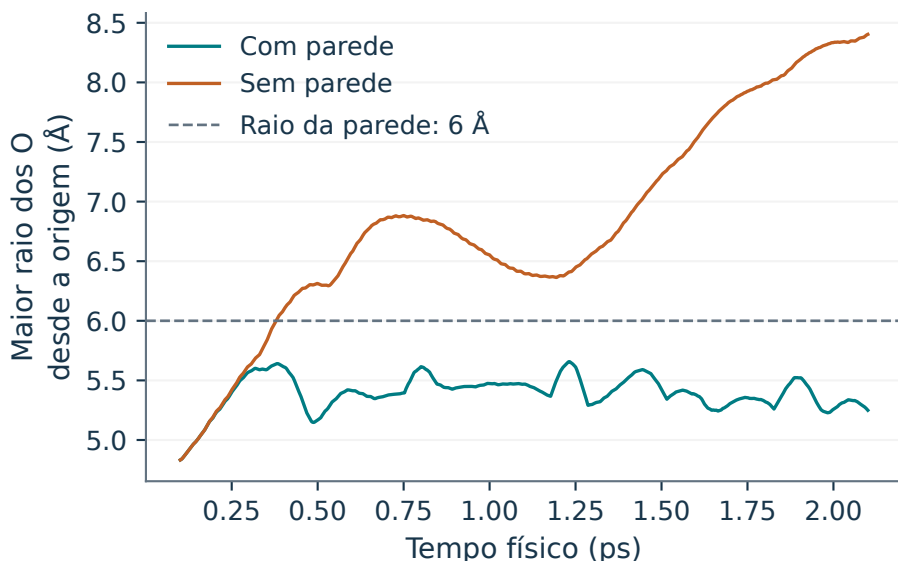
Figura 7.2: Distâncias radiais dos O à origem nos controles com e sem parede. A referência de 6 Å pertence a esse raio, não à distância Zn–O.
