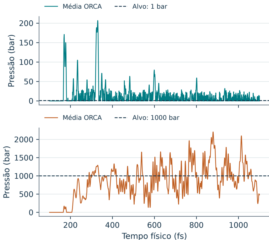
Figura 10.2: Pressão média da parede registrada pelo ORCA nos dois ramos de C2. As linhas horizontais, diferenciadas por traço, são os alvos externos de cada painel. A pressão medida é distinta do alvo.
