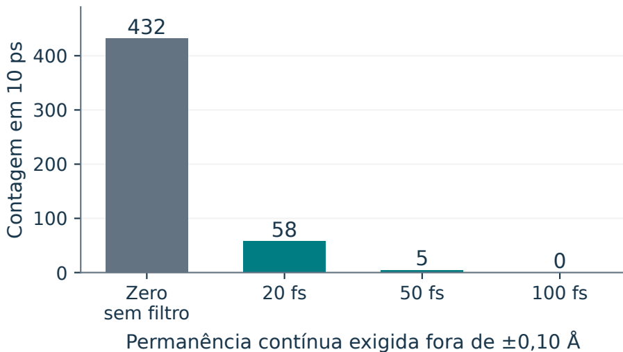
Figura 9.3: Contagens da referência inteira de 10 ps: 432 cruzamentos de zero versus mudanças com permanência contínua de 20, 50 ou 100 fs fora da banda central.
