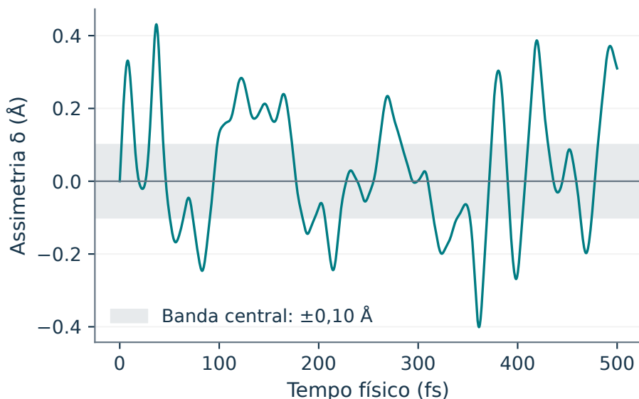
Figura 9.1: Zoom dos primeiros 500 fs de \text{H}_5\text{O}_2^+ XTB2/CSV. A coordenada delta distingue o O mais próximo, e a banda central tem limites de menos e mais 0,10 Å.
