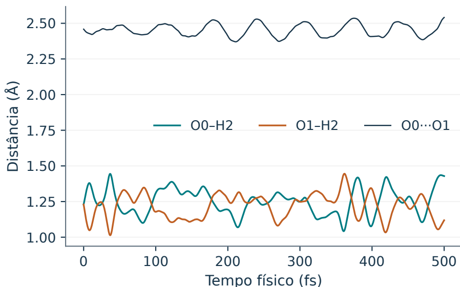
Figura 9.2: Distâncias O0-H2 e O1-H2 no mesmo zoom de 0–500 fs. Sua comparação dá o sinal de delta sem mudar a identidade do H acompanhado.
