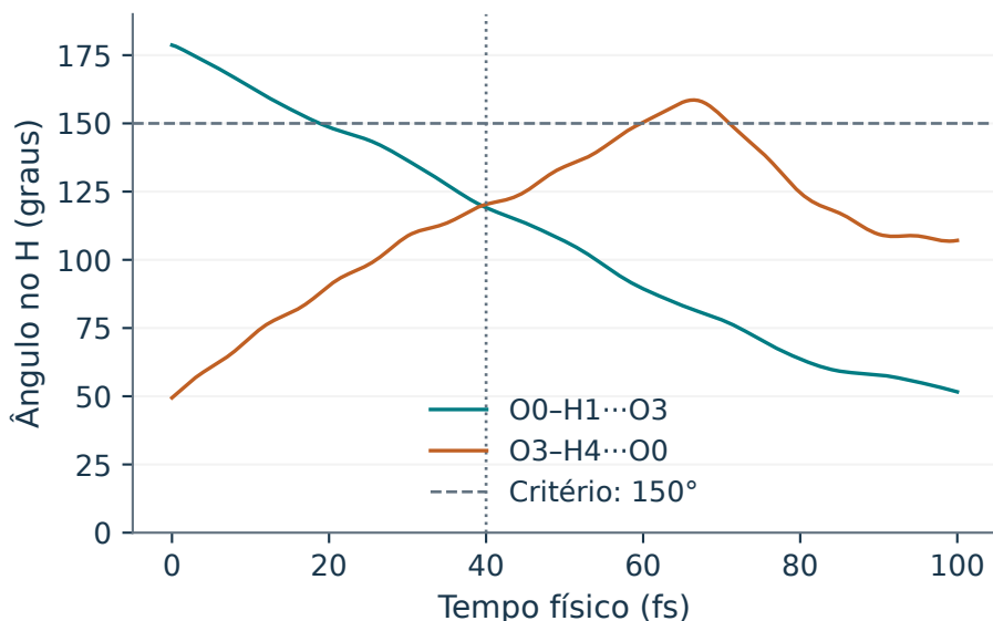
Figura 3.2: Zoom de 0–100 fs dos ângulos O–H...O e referência angular de 150 graus. Proximidade e orientação devem ser avaliadas juntas.
