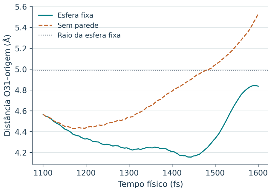
Figura 10.3: C3: distância de O31 à origem nos dois ramos, de 1100,5 a 1600 fs. O31 identifica a mesma água externa em ambos. A linha horizontal mostra o raio da esfera mantida no ramo fixo; no ramo None não existe parede.
