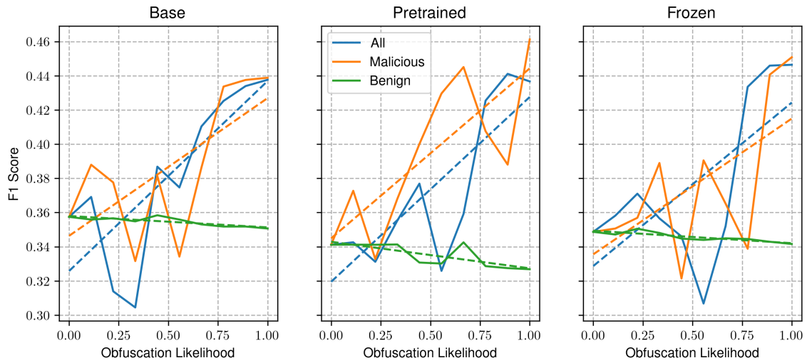
(b) Sequence level F1 score
