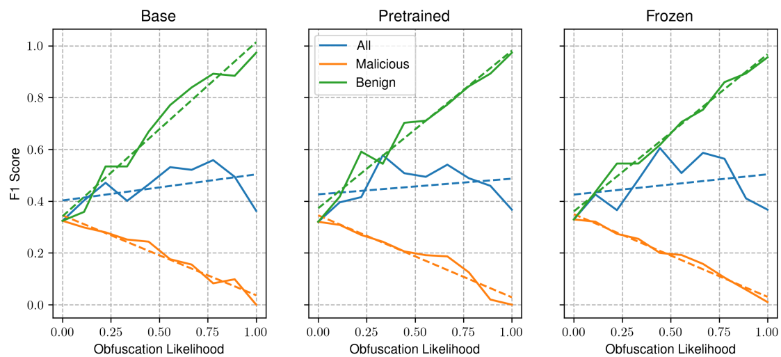
(a) File-level F1 score
