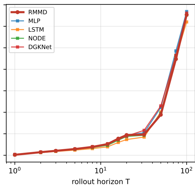
AUGD
