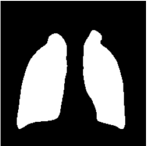
Pred Mask
