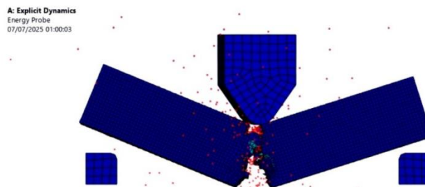
Gambar 4. 23. Visualisasi Energi Internal
