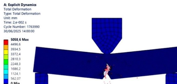
Gambar 4. 1. Visualisasi Total Deformasi
