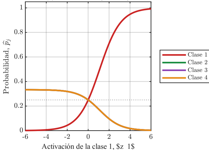
(b) Función \text{softmax}
