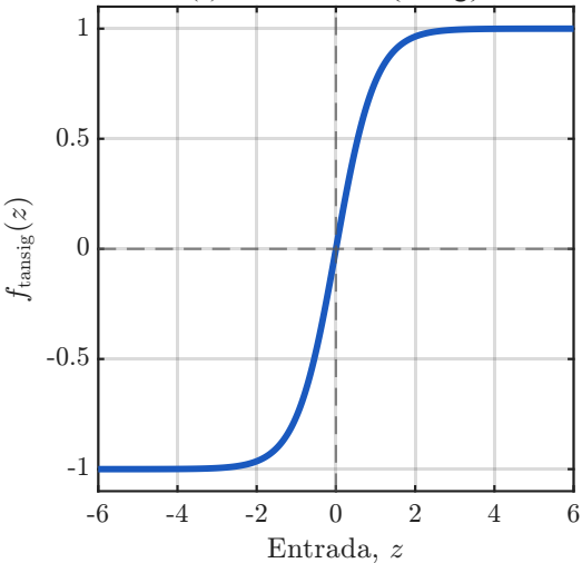
(a) Función \text{tansig}
