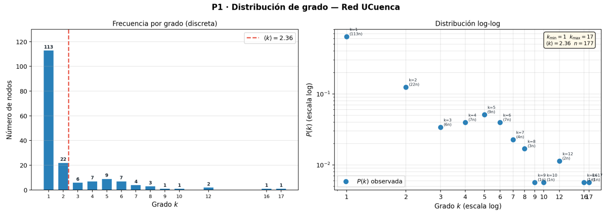
(a) Distribución de grado P(k) en escala log-log.
