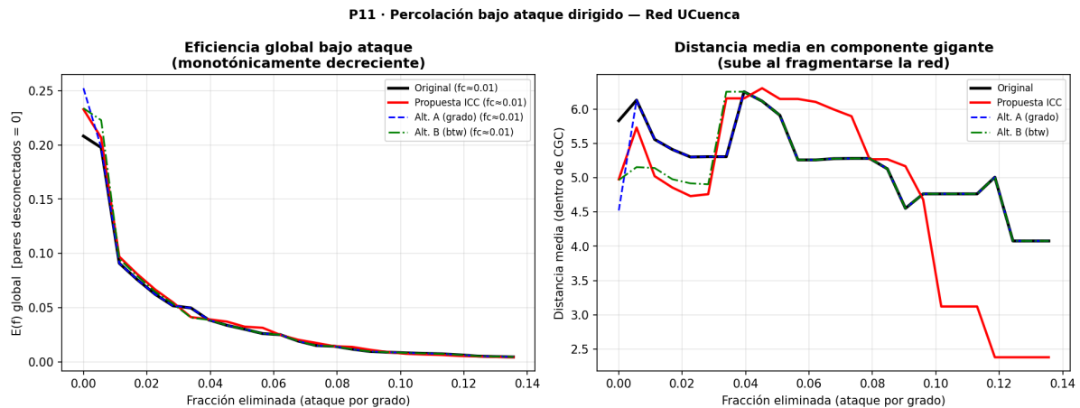
Fig. 20. Percolación bajo ataque dirigido. Izquierda: eficiencia global sobre todos los pares originales (pares desconectados = 0, curva monótonicamente decreciente). Derecha: distancia media dentro de la componente gigante restante.
