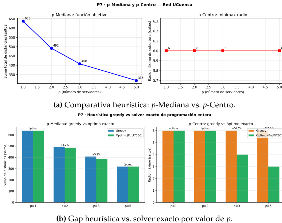
Fig. 12. Localización de instalaciones: modelos y comparativa de métodos.
