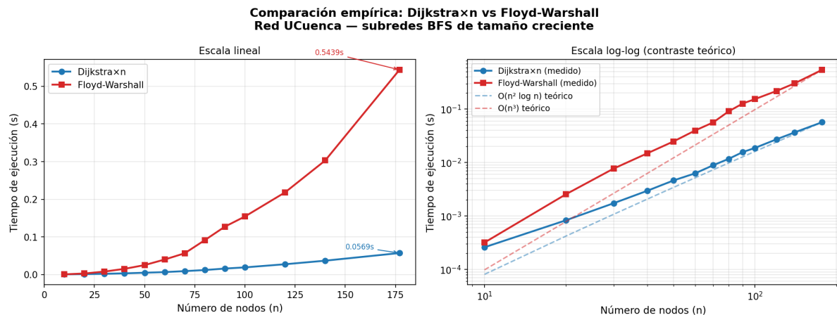
(a) Tiempo de ejecución vs. tamaño de la red.
