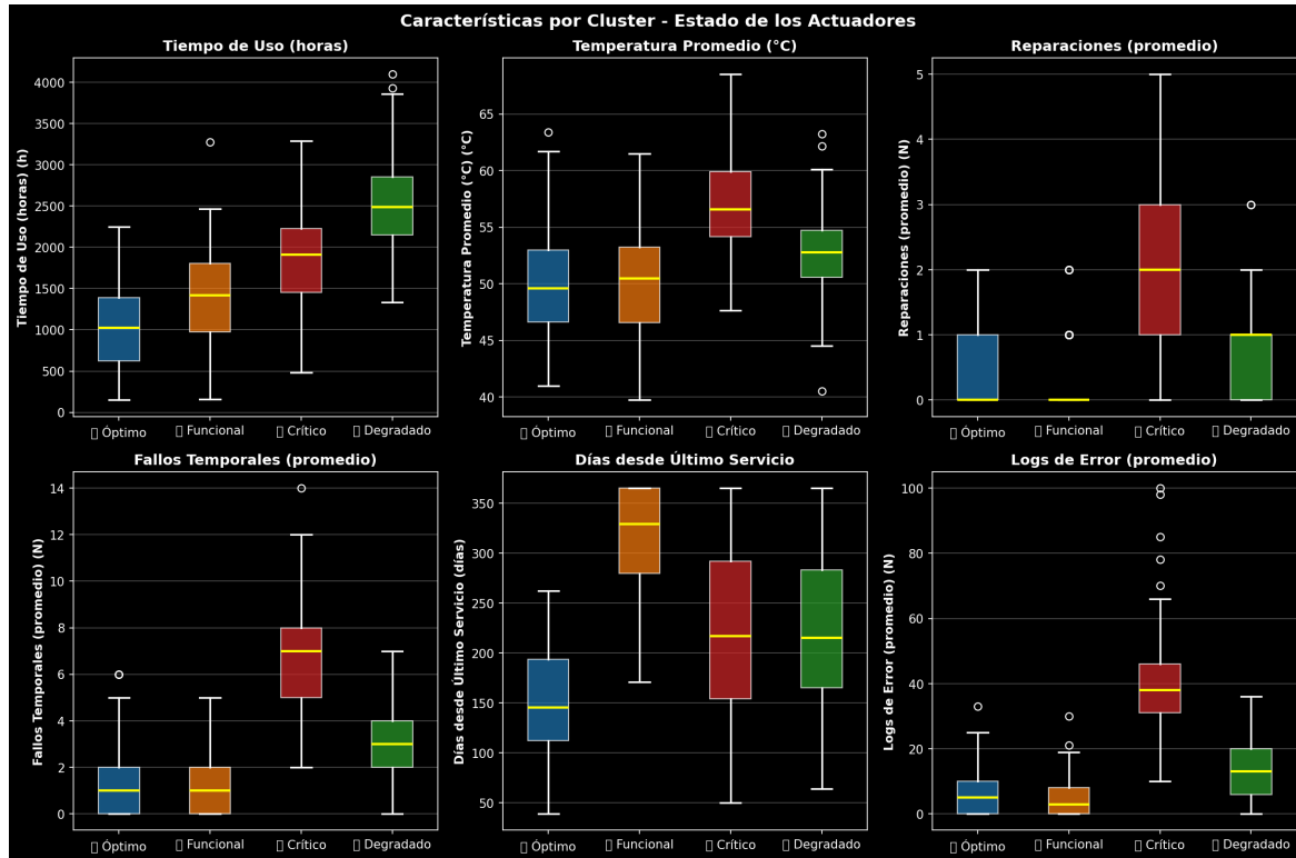
Figura 3: Estadísticas Clusters
