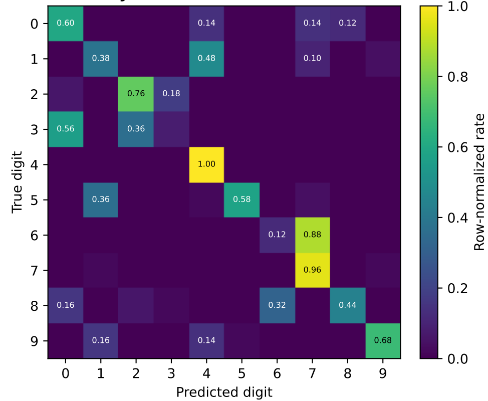
(d) Test confusion Accuracy = 0.560
