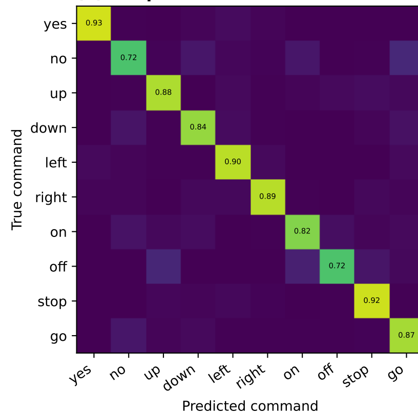
(d) Temporal EGFN test confusion
