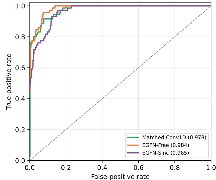
(b) Test ROC
