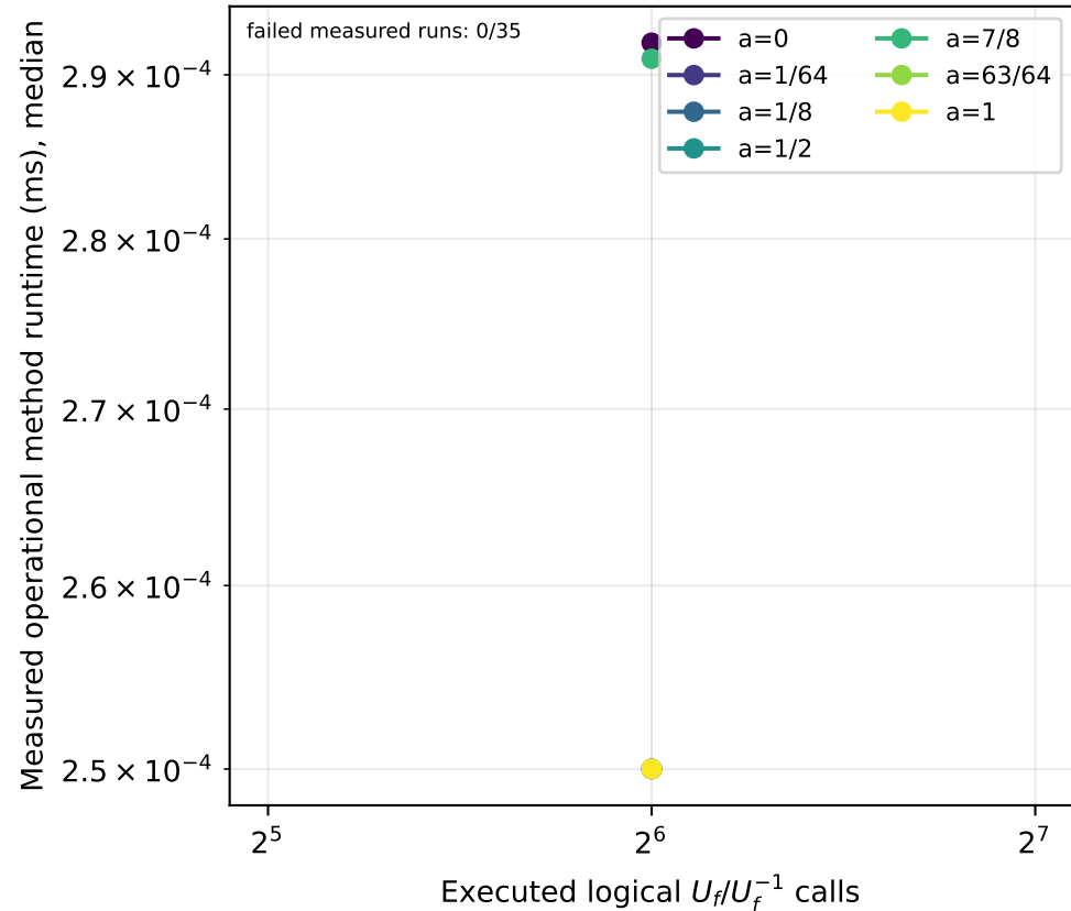
Exact enumeration
