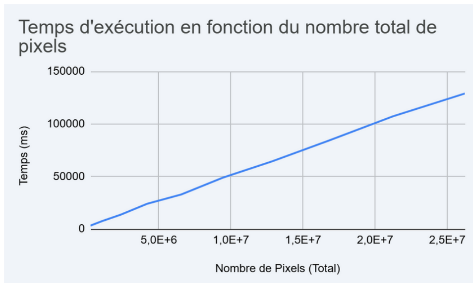
FIGURE 1 – Temps d'exécution en fonction des pixels
