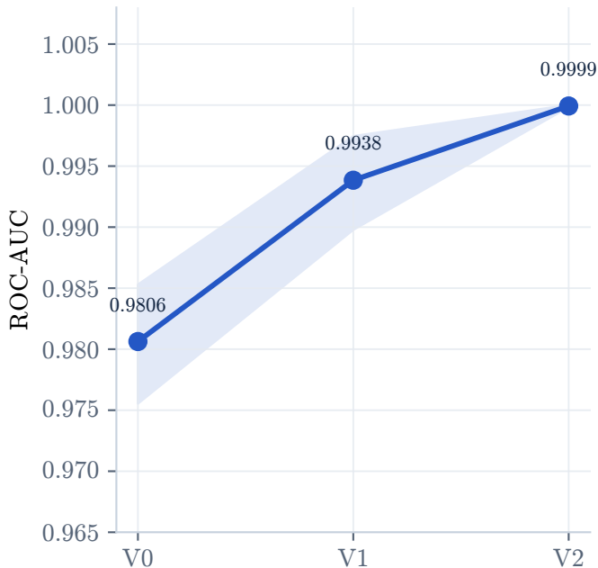
ROC-AUC
