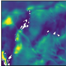
ResUNet++
