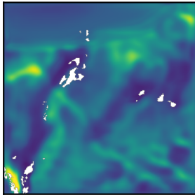
U-Net
