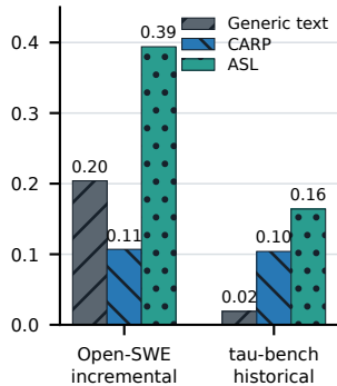
C Agent state raises F1
