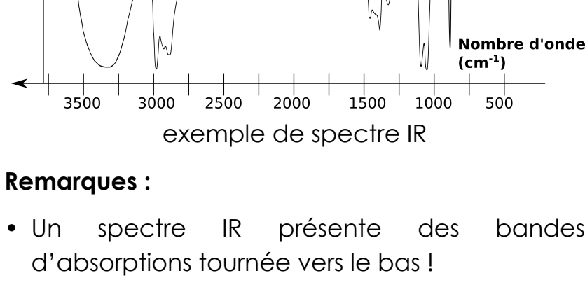
exemple de spectre IR
