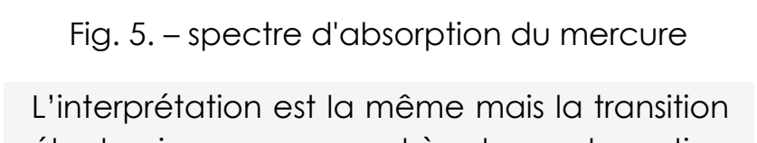
Fig. 5. – spectre d'absorption du mercure
