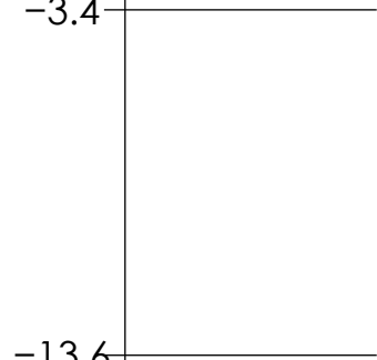
Fig. 2. – Niveaux d'énergies de l'atome d'hydrogène
