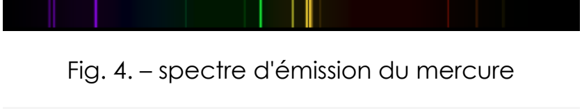
Fig. 4. – spectre d'émission du mercure
