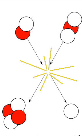
Fig. 2. – Fusion nucléaire
