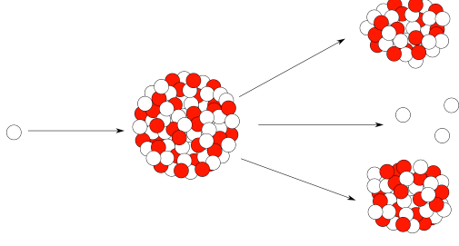
Fig. 3. – Fission nucléaire
